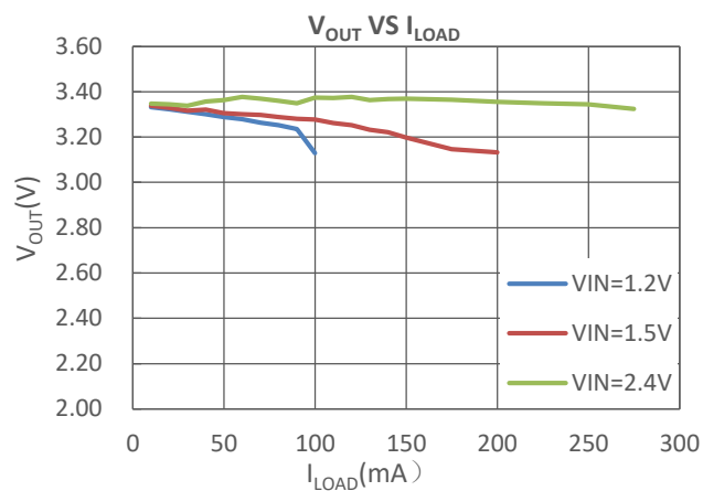
图 1. V_{OUT} VS I_{LOAD} ( L=22\mu H )
